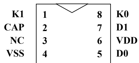
TTP277-A08N 8-SOP-A
