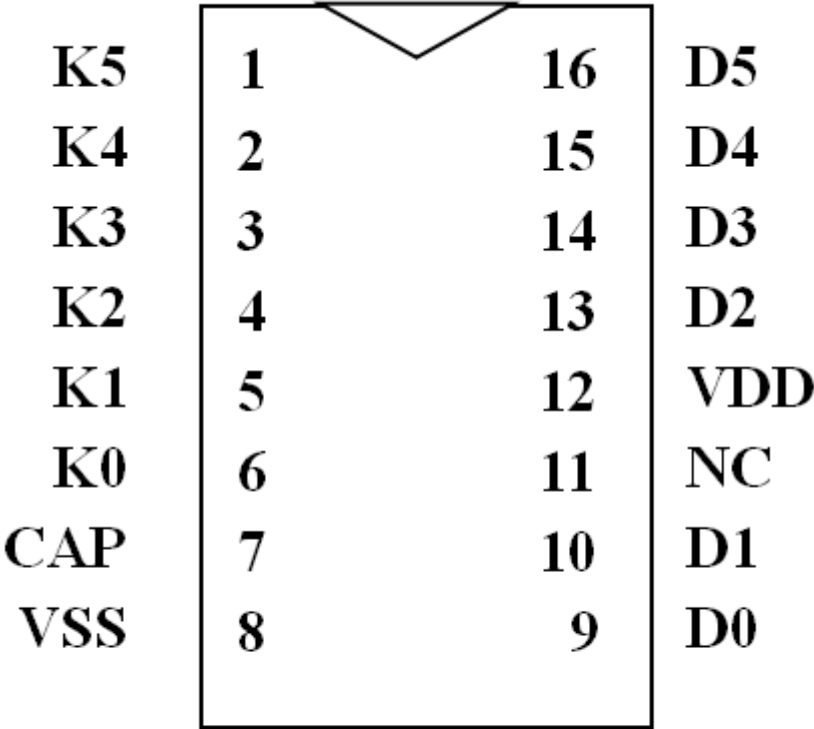
TTP272-AOBN 16-SOP-A
