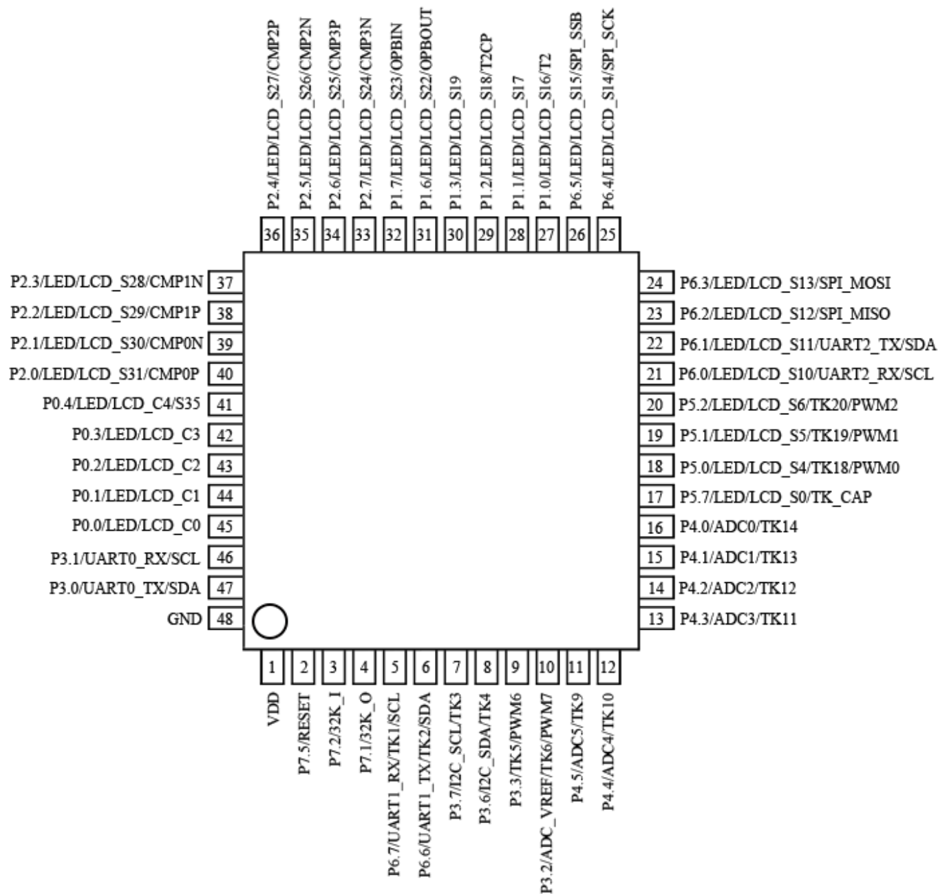
图 5-1-2LQFP48 封装图
