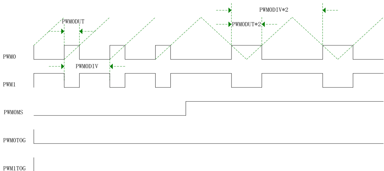
图 21-1-4 PWM0、PWM1 输出互补波形
