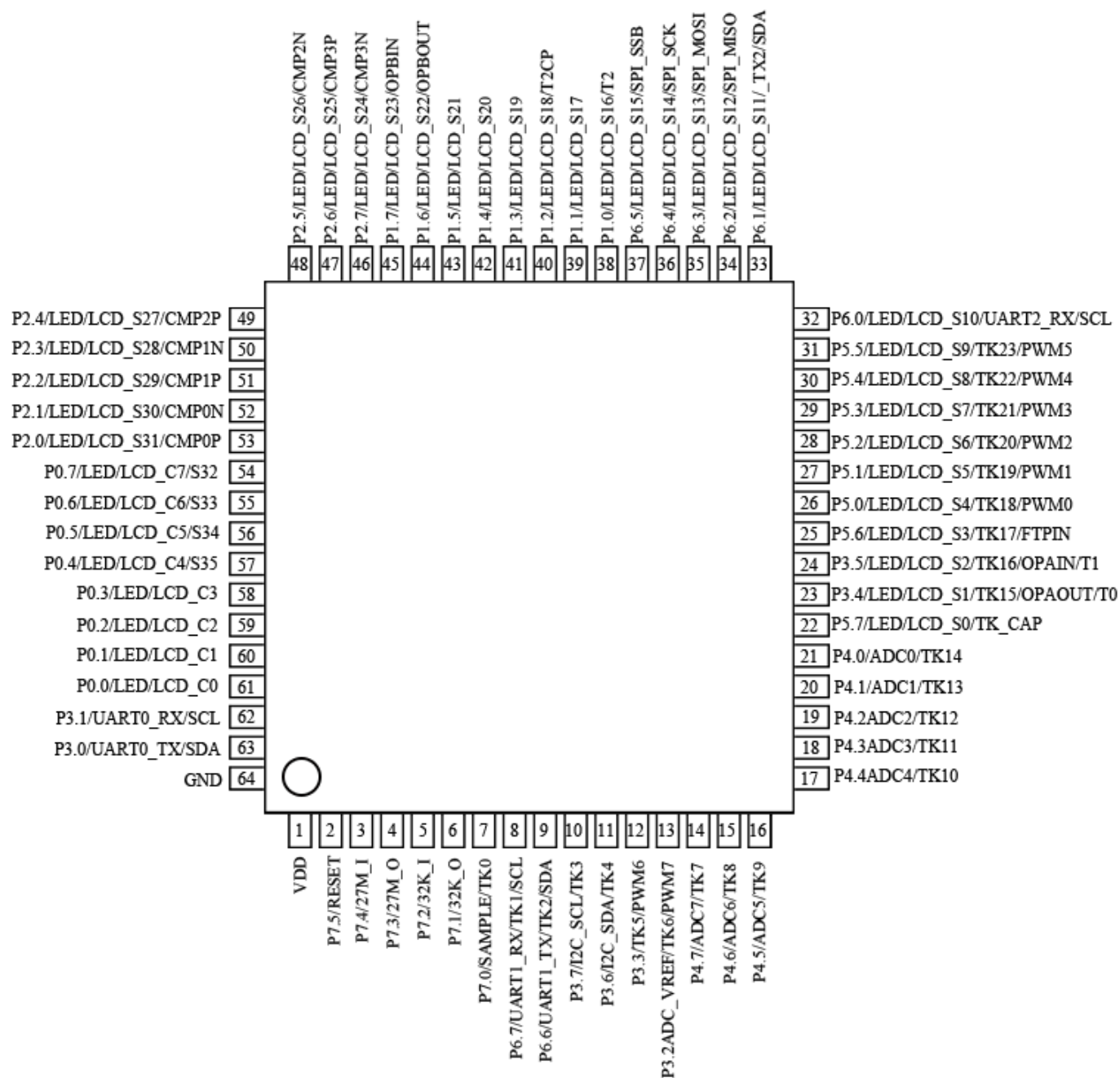
图 5-1-1 LQFP64 封装图
